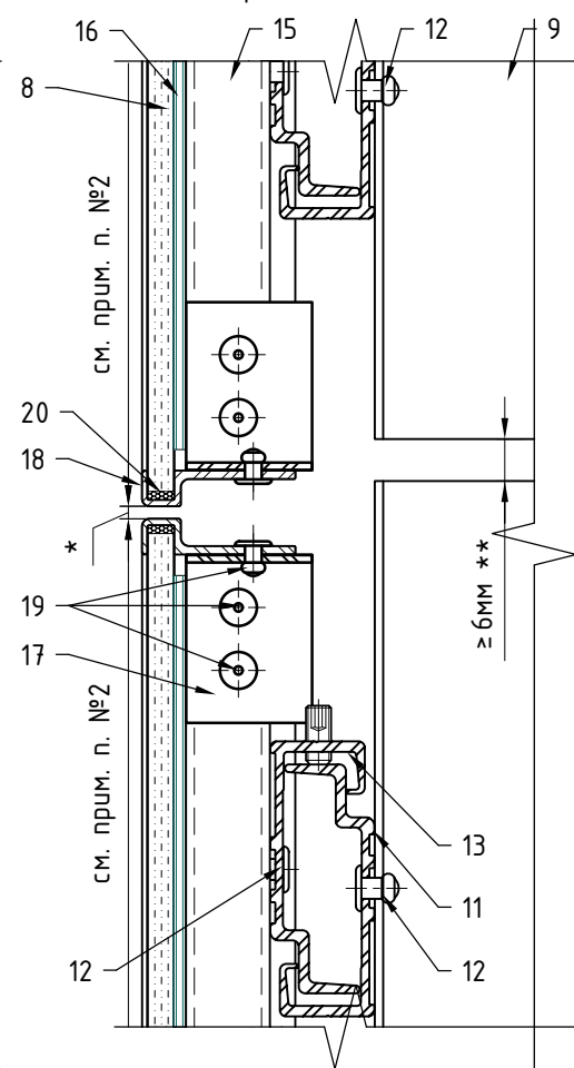
Фрагмент №1 (вариант тех.решения, где длина аграрного профиля и его положение задаются габаритами кассеты)
