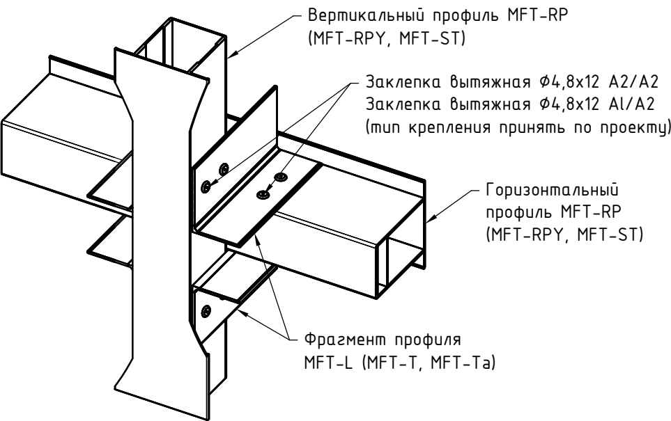
Узел №4 (увеличено)
