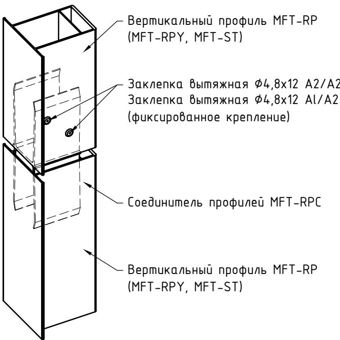
Узел №6 (увеличено)
