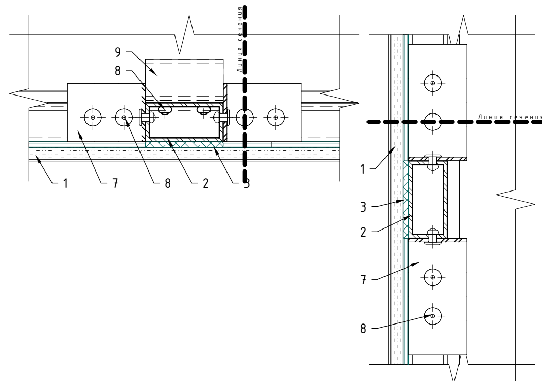
Узел №2 (соединение элементов каркаса, увеличено)
