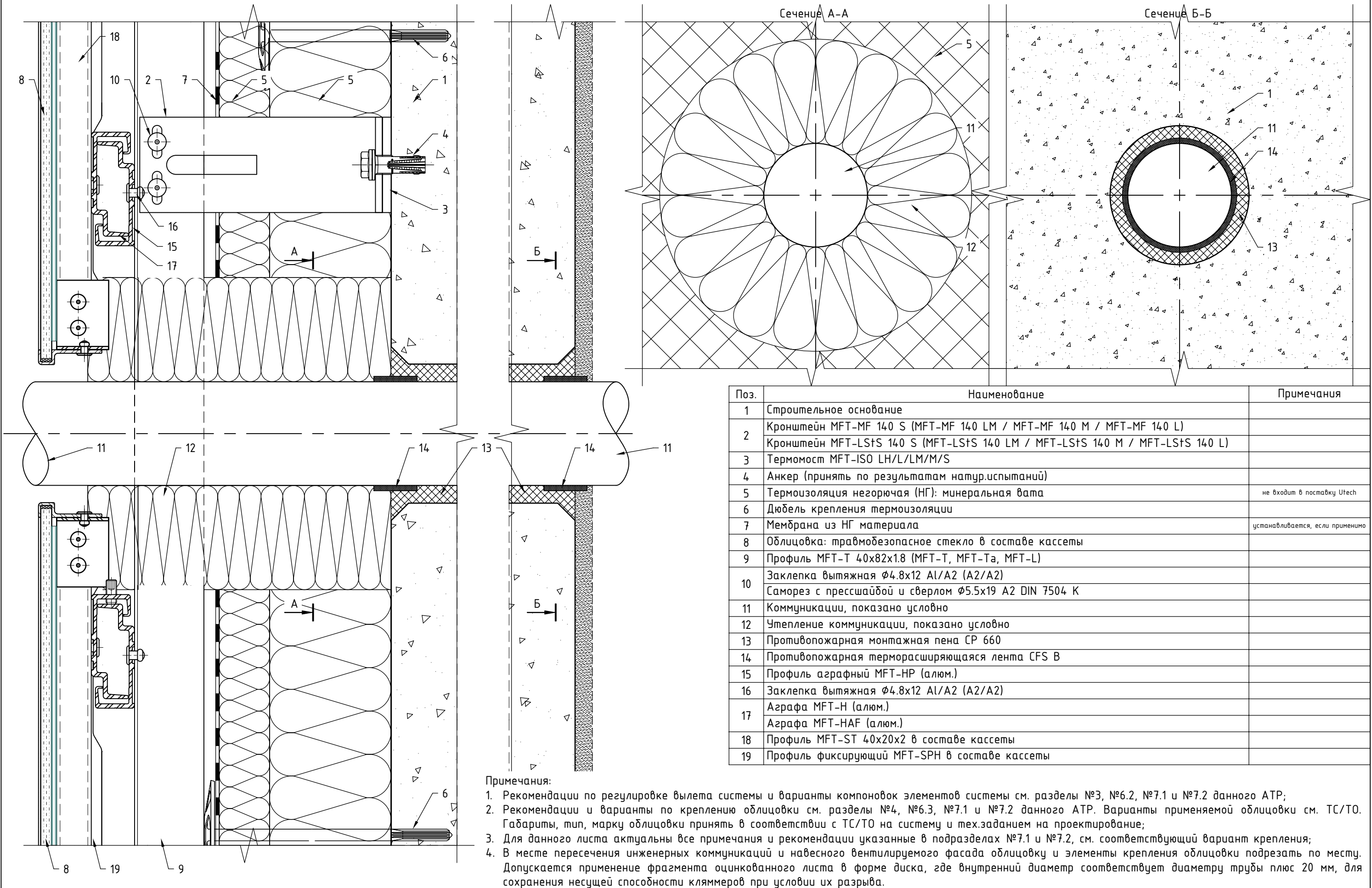
7.11. Ввод коммуникаций: элементы "Light", скрытое крепление на аграфы.
