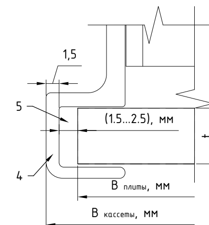
Узел №Б (увеличено)
