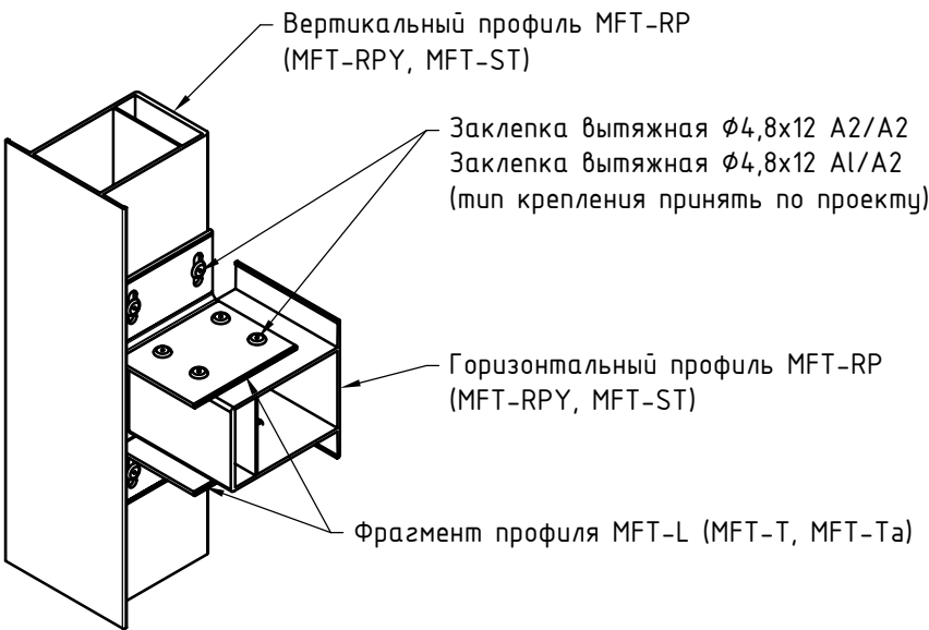
Узел №5 (увеличено)
