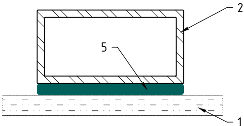
Приклеивание стекла к профилю MFT-ST: после приклеивания
