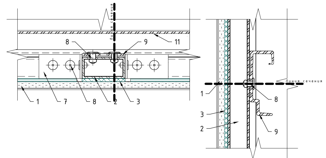
Узел №1 (установка аграф, увеличено)
