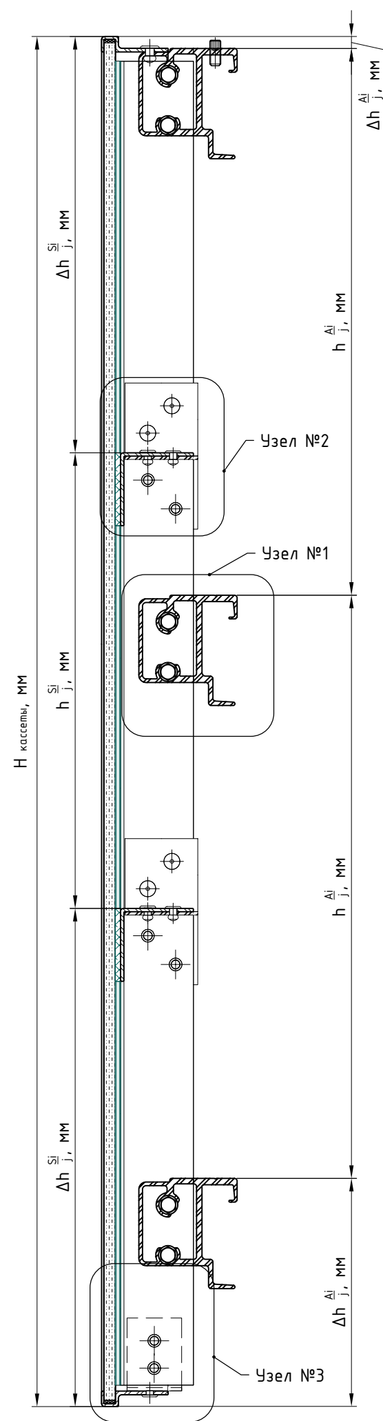
Сечение 4-4
