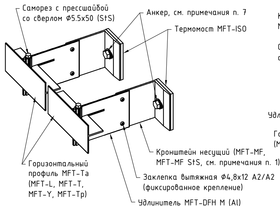
Узел 1 (увеличено)
