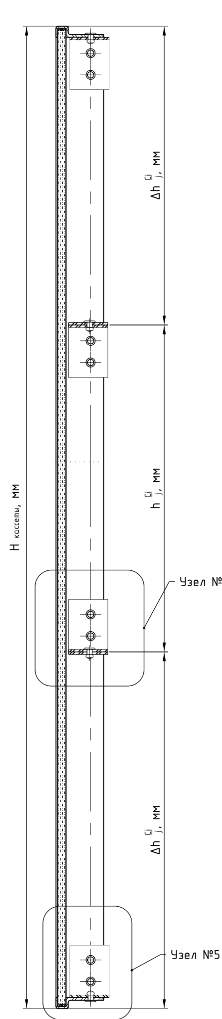
Сечение 5-5
