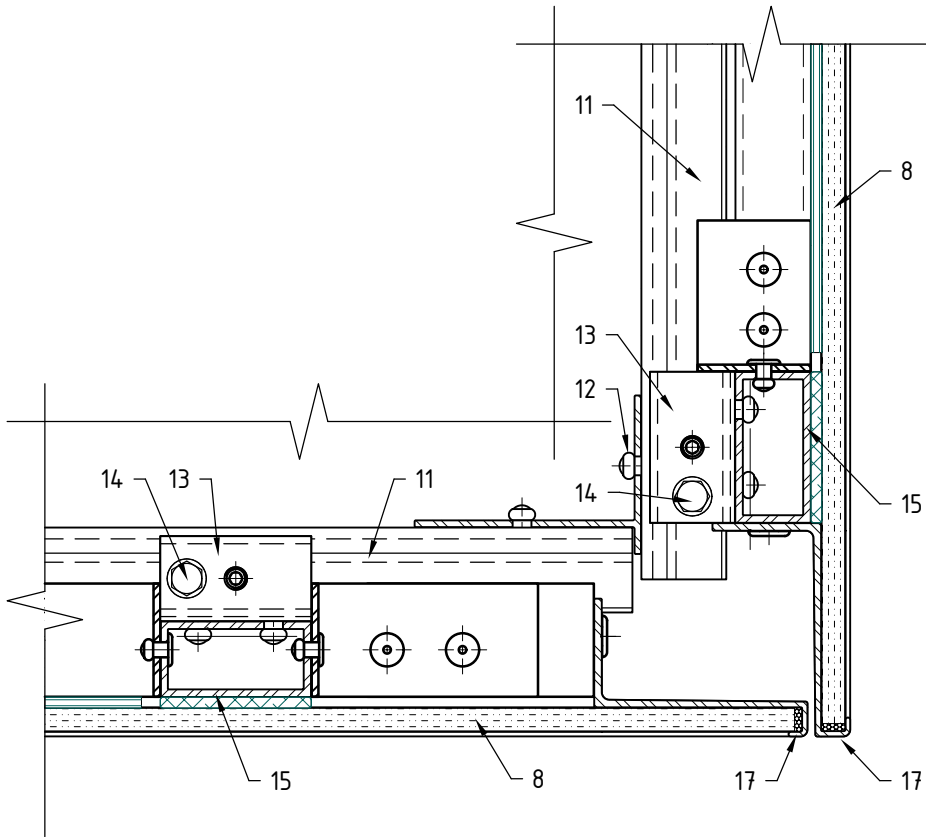
Фрагмент №1: в уровне крепления кассеты к направляющим.
