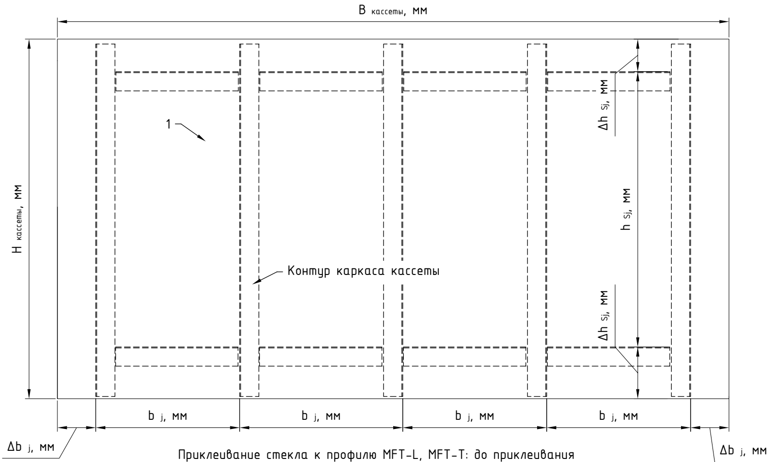
Горизонтальная ориентация плит облицовки (плита показана с лицевой стороны)
