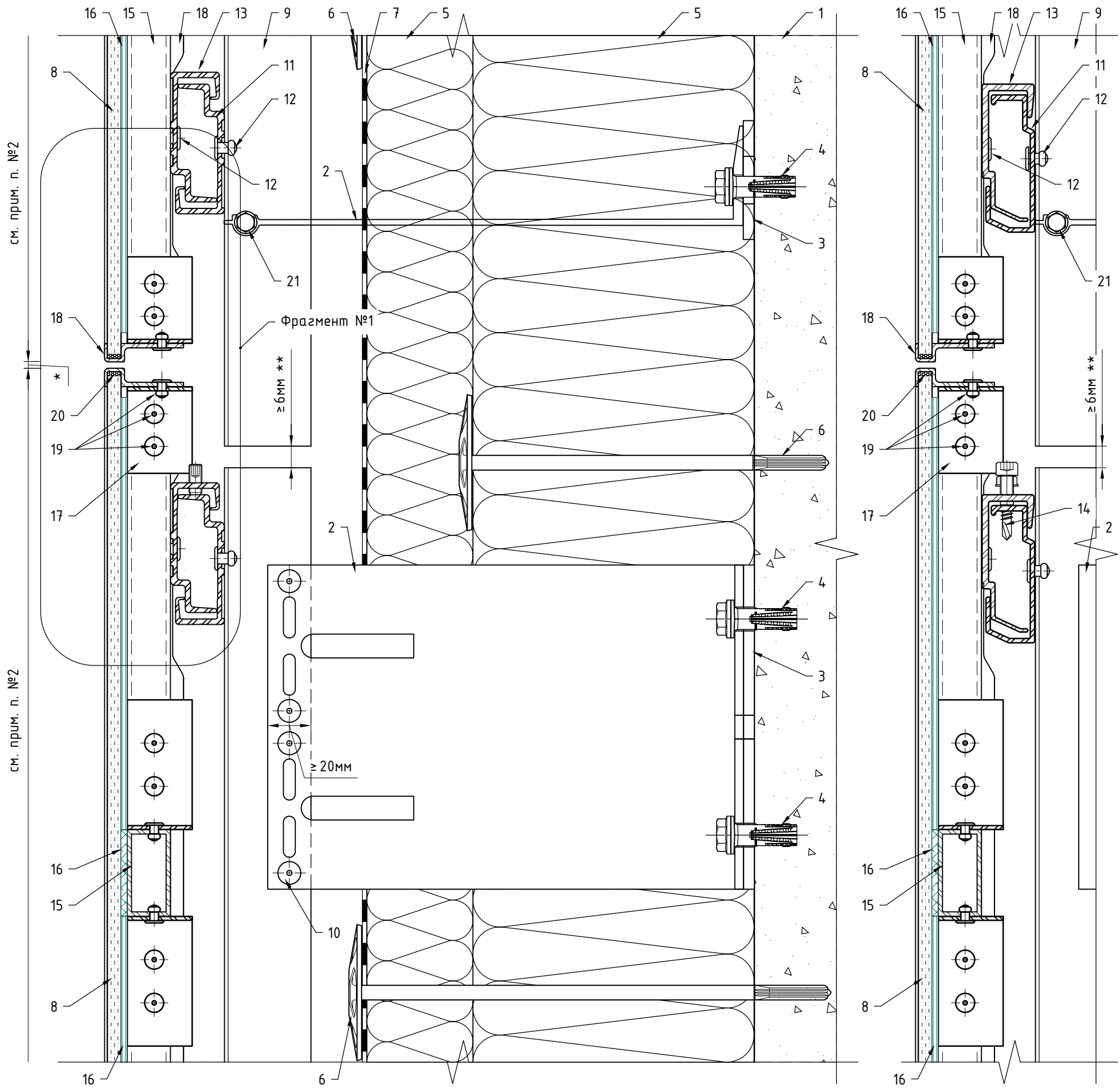
Фрагмент №1 (показано для аграр типа E)
