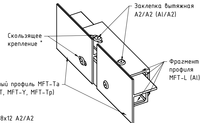
Фрагмент узла стыковки гор.направляющей ** (увеличено)
