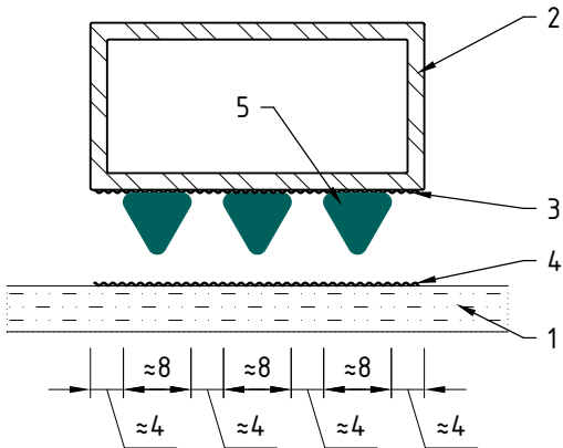
Приклеивание стекла к профилю MFT-ST: до приклеивания
