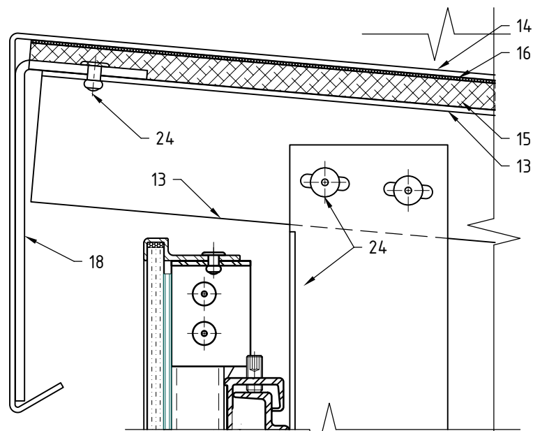
Вариант крепления парапетной крышки №3
