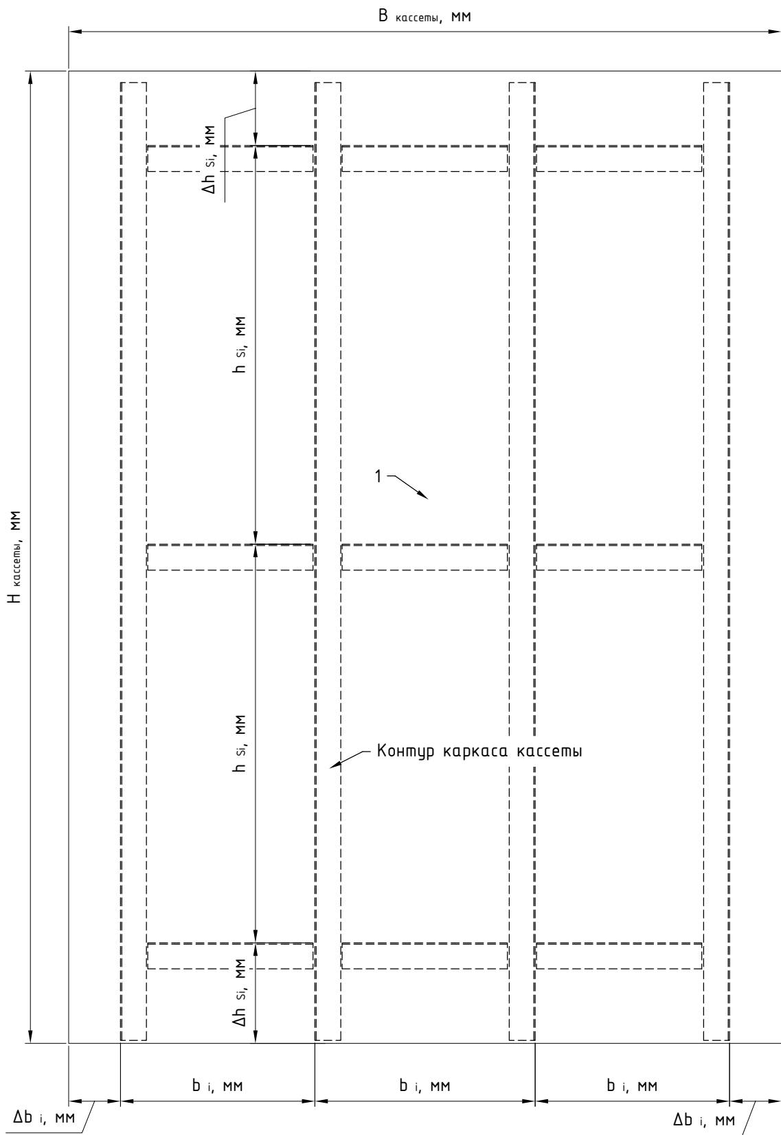
Вертикальная ориентация плит облицовки (плита показана с лицевой стороны)
