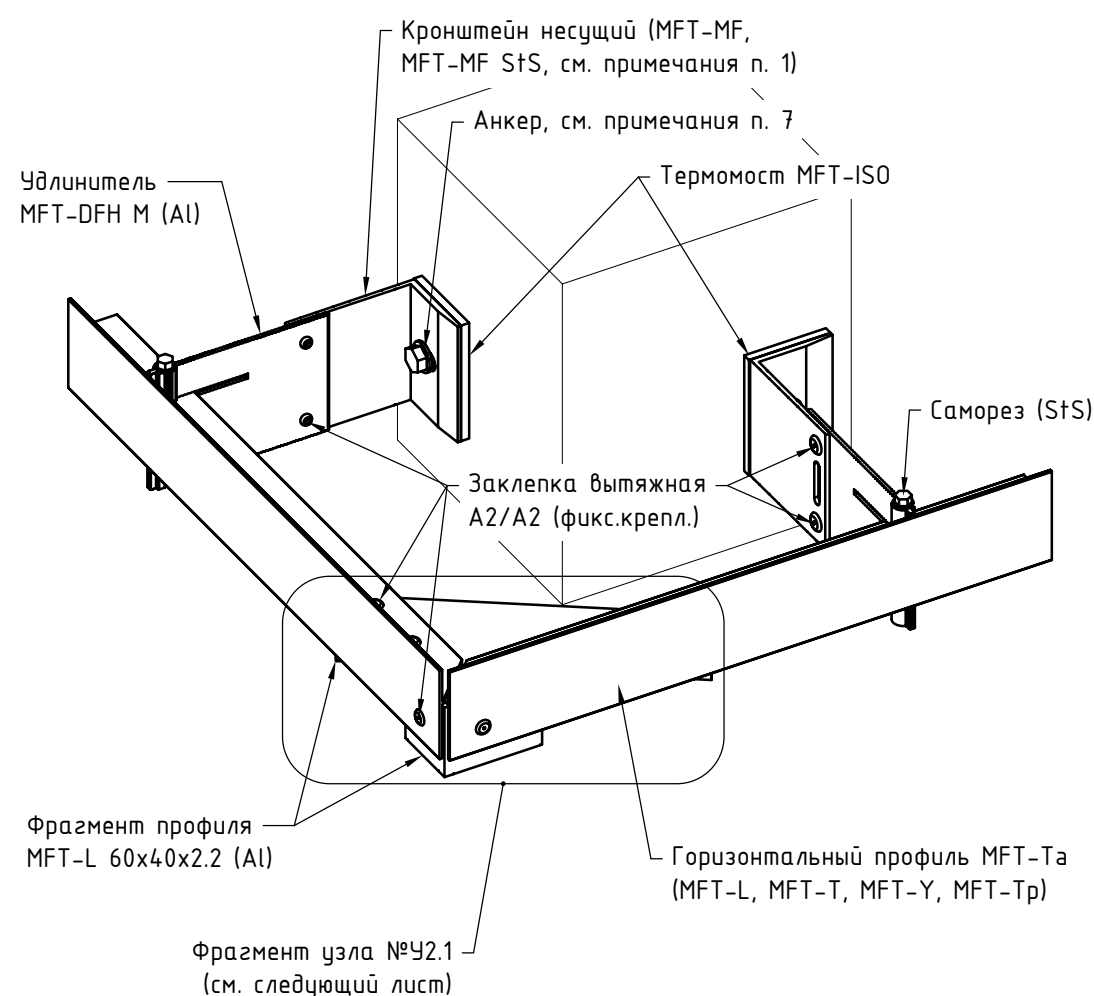
Узел 2 (увеличено)
