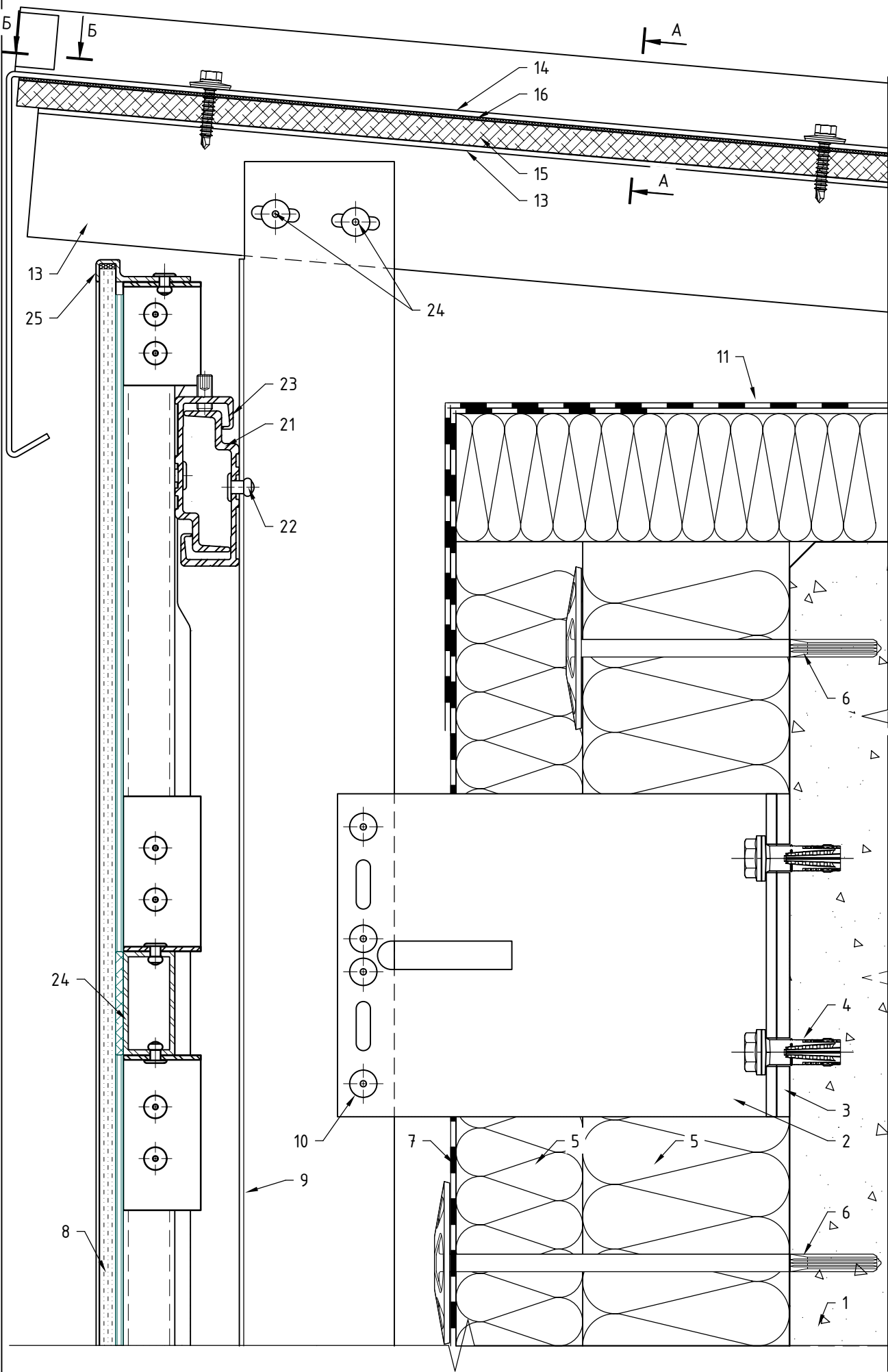
7.9. Примыкание к парапету: элементы "Light", скрытое крепление на аграфы.
