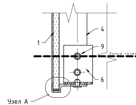
Узел №5 (фиксация профиля MFT-SPH к элементам каркаса, увеличено)
