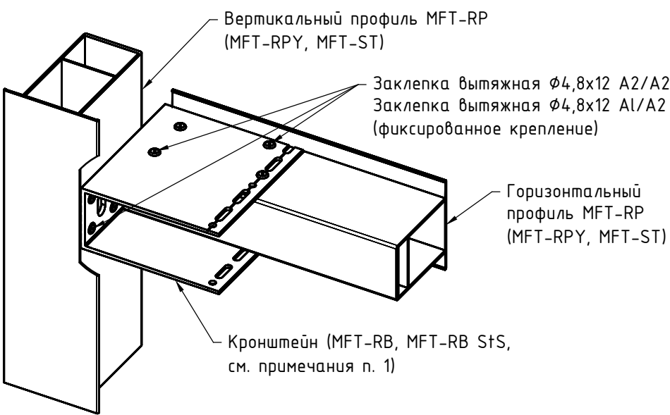
Узел №3 (увеличено)
