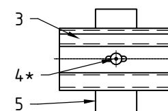
Крепление горизонтального профиля к вертикальной направляющей с шириной полки \leq 45\text{мм}
